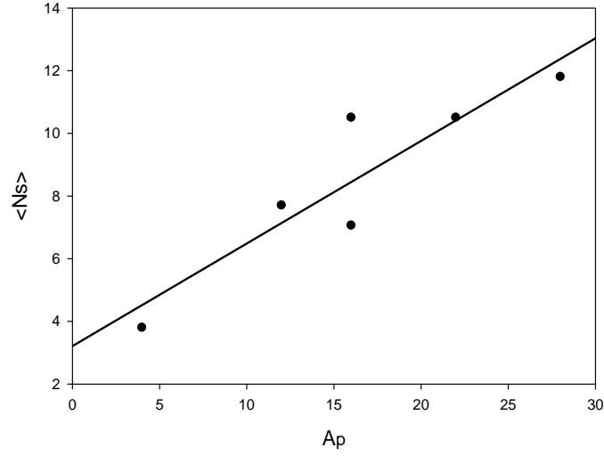
الشكل (3) يوضح العلاقة بين متوسط الجسيمات الرذاذية وعدد الكتلة للقذيفة
