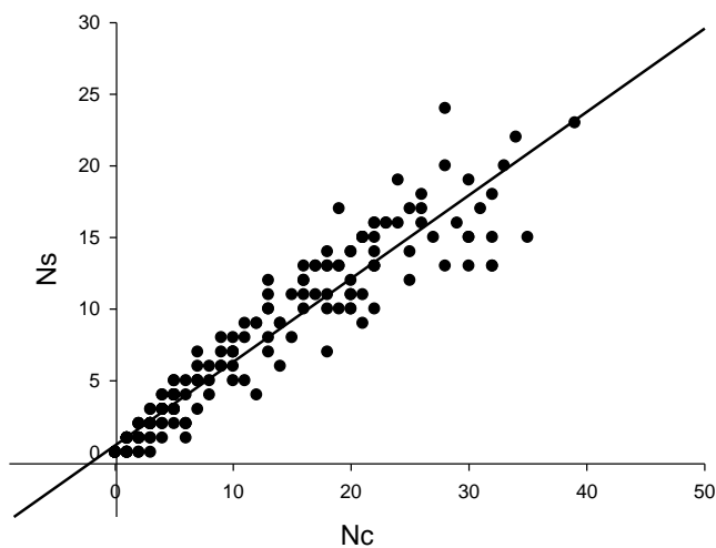
الشكل (9) يوضح العلاقة بين التعددية المركبة و الجسيمات الرذاذية
