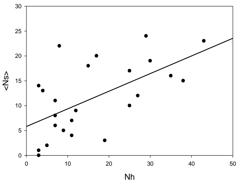
الشكل (6) يوضح العلاقة بين تعددية الجسيمات كثيفة التأين و متوسط الجسيمات الرذاذية
