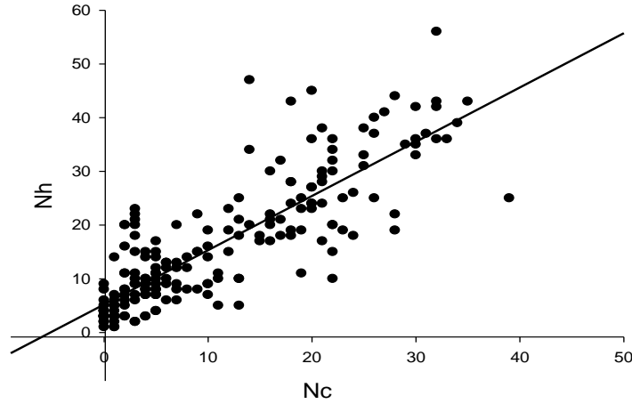
الشكل (12) يوضح العلاقة بين التعددية المركبة و الجسيمات كثيفة التآين
