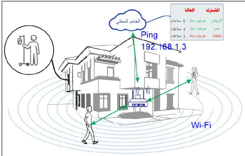
شكل 11: مخطط منظومة التواجد داخل المنزل.
