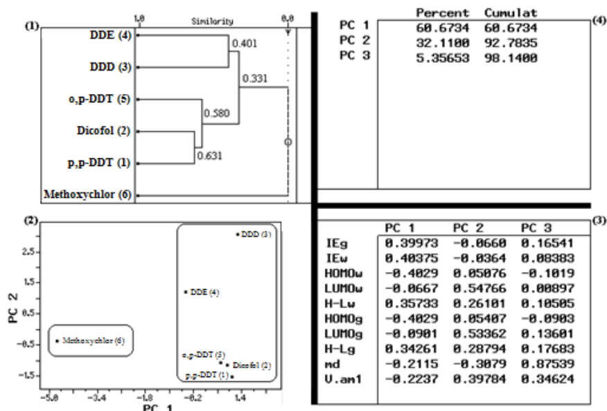
شكل (2): يوضح التحليل الكيمومتري (PC1 و PC2) لبعض قيم الخصائص الفيزيوكيميائية المحسوبة لمجموعة الـ p,p-DDT المحرمة
