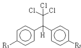
شكل (3): يوضح البنية الكيميائية للمركبات المتماثلة لمركب p,p DDT
