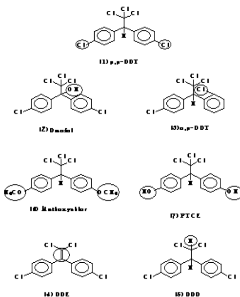
شكل (1): يوضح مركبات مجموعة الـ (p,p'-DDT: 1,1,1-trichloro-2,2-dichlorophenyl) ethane)
