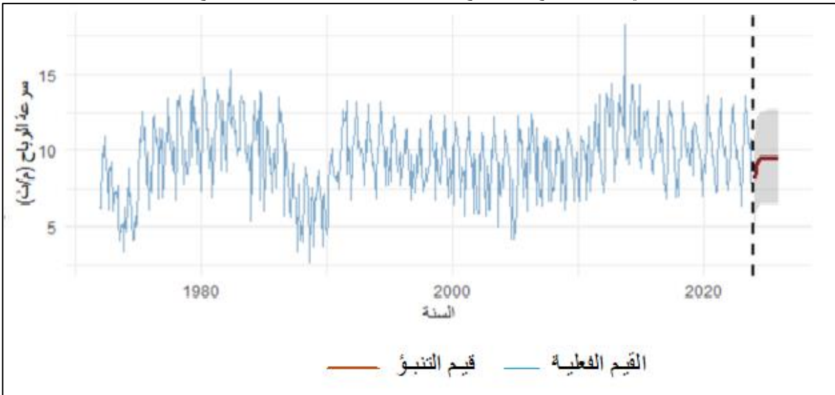
الشكل (4) المنحنى الزمني باستخدام النموذج الهجين للقيم الفعلية والتنبؤات، مع منطقة فترة الثقة الرامدية
