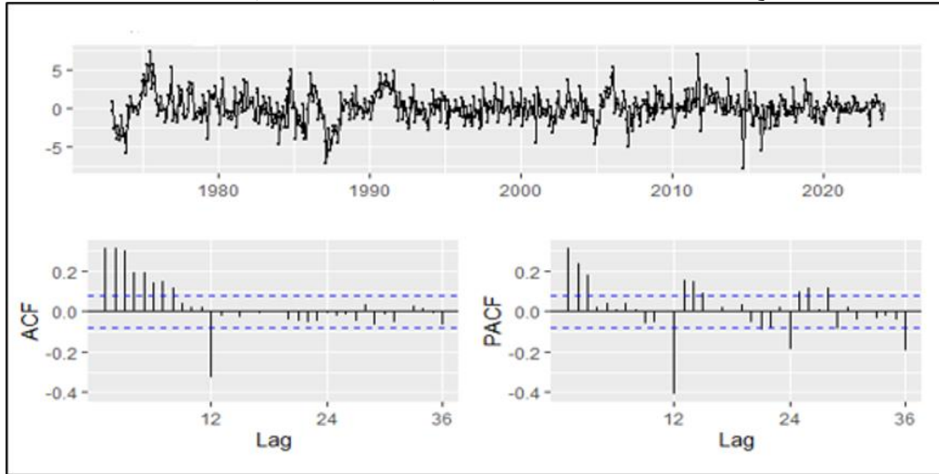
الشكل (3): معاملات الارتباط الذاتي والارتباط الذاتي الجزئي لسرعة الرياح الشهرية في منطقة سبها للفترة 1972-2023.
